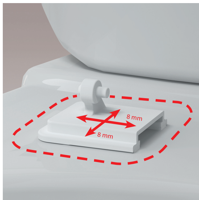
A pántok beállításának széles változatai lehetővé teszik az ülőkék optimális felszerelését különböző típusú WC-csészékre.
